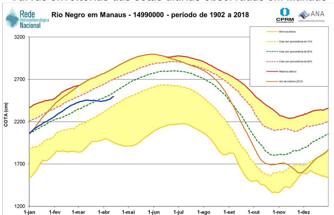
Gráfico 01: Cotagrama do Rio Negro em Manaus. Cota em 13/04/2018: 24,99 m
