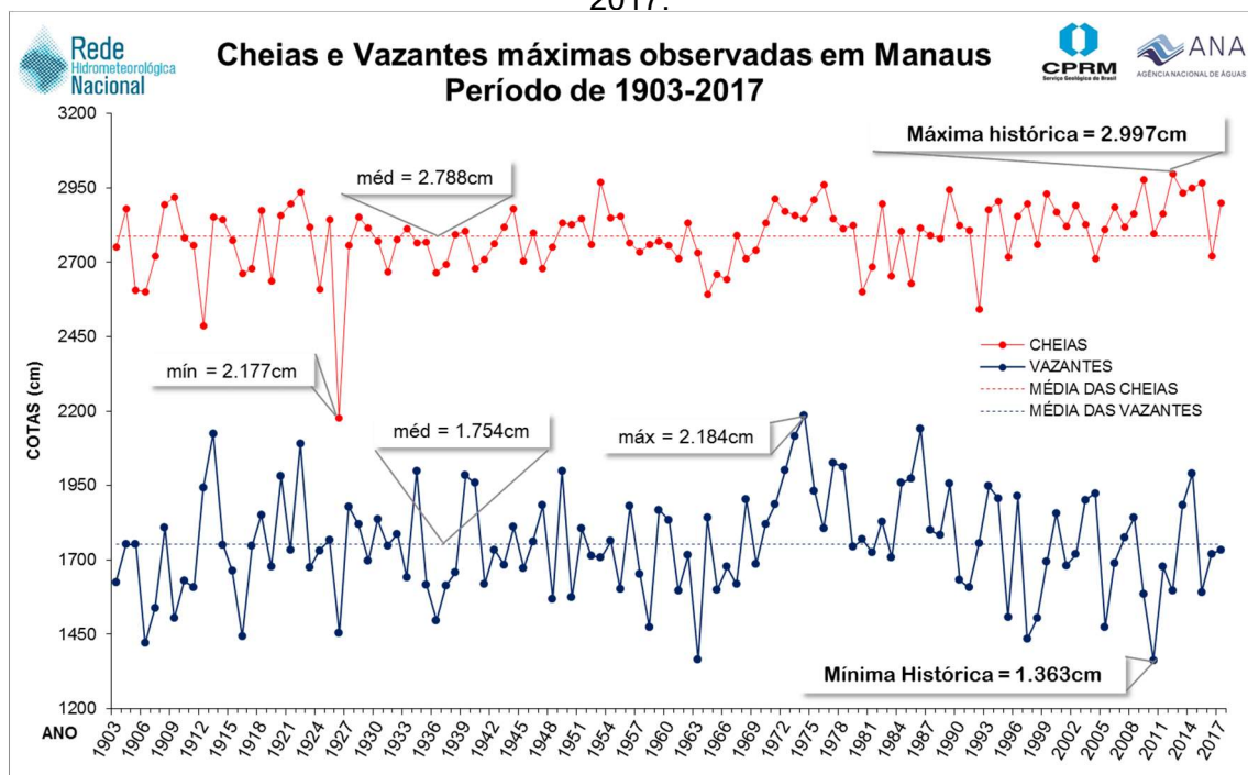
Gráfico 03: Dados de cotas máximas e mínimas anuais observadas em Manaus no período 1902 – 2017.
